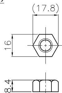
ナット (2ヶ)
