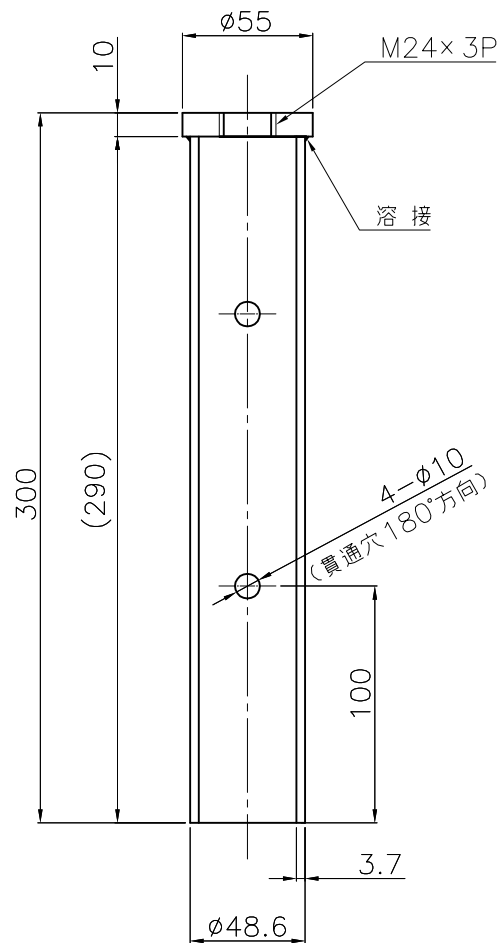
ネジ付鋼管
