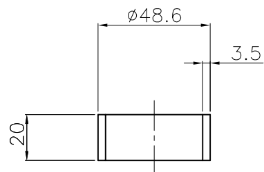
スペーサ
