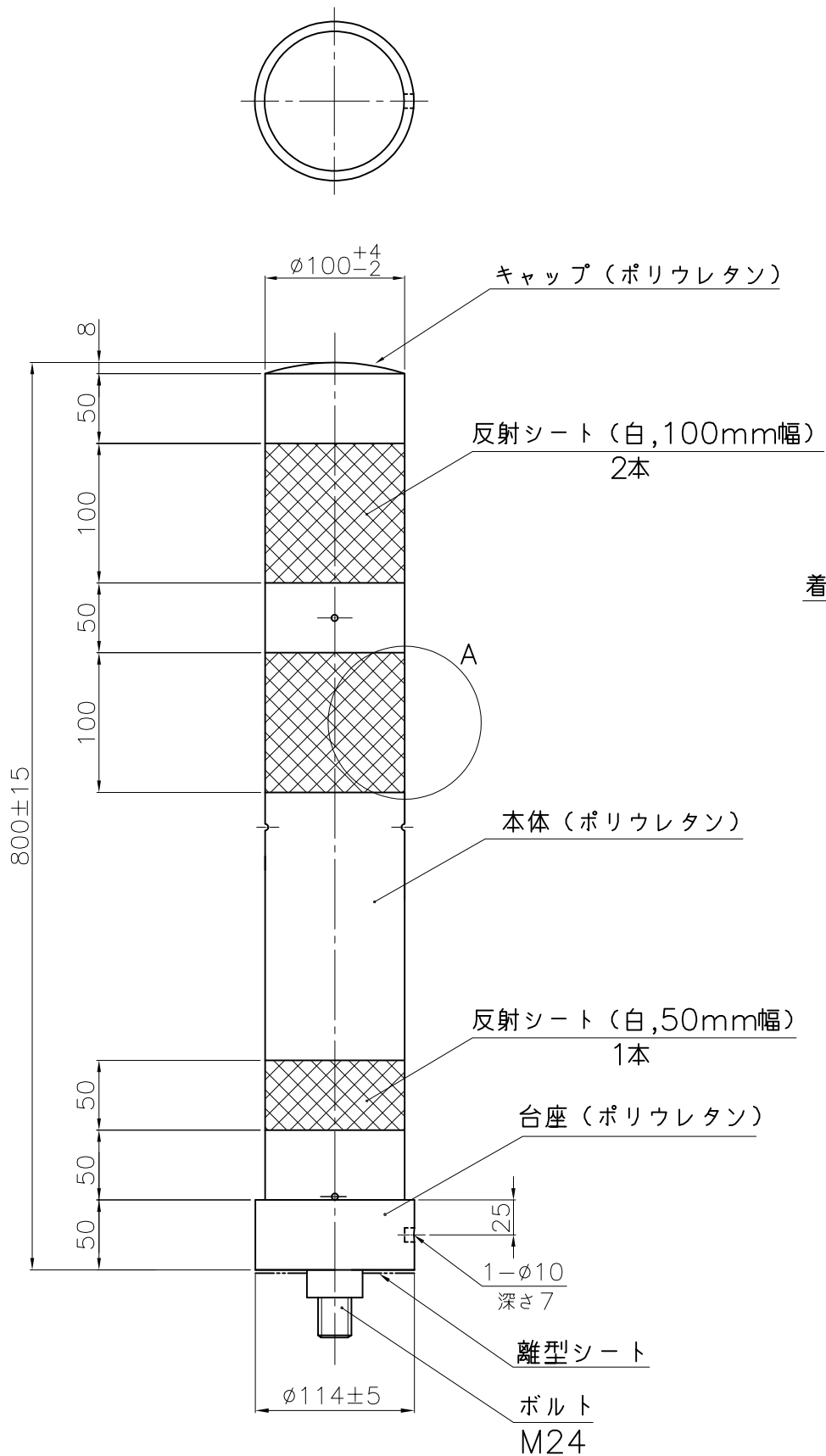
埋設用脚セット図
