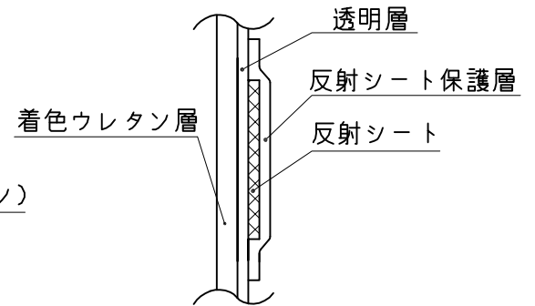
A部詳細断面図
