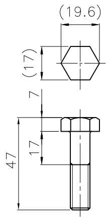
ボルト (M10X1.25P)
