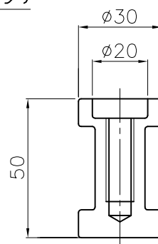
埋設用脚
