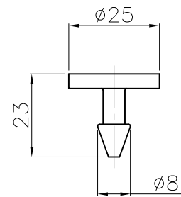
抜止メピン
