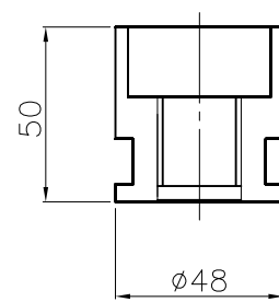
埋設用脚
