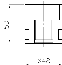
埋設用脚
