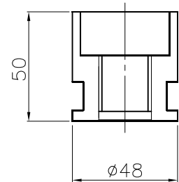
埋設用脚
