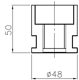
埋設用脚
