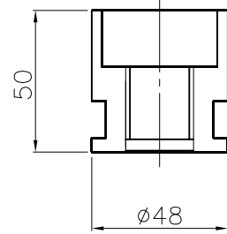
埋設用脚
