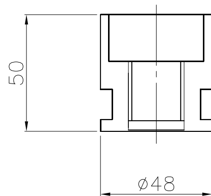
埋設用脚
