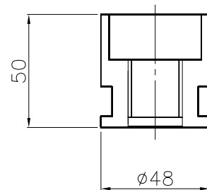
埋設用脚
