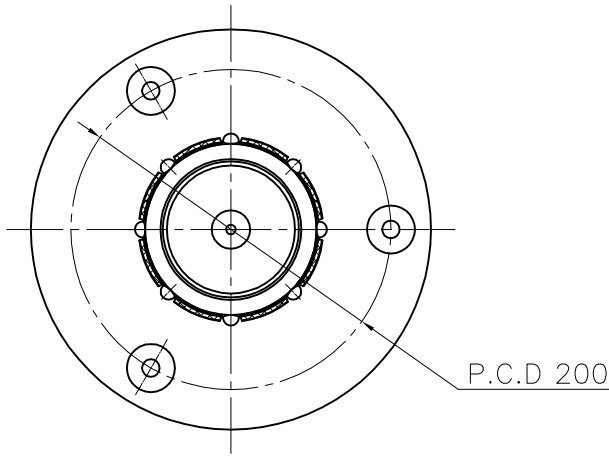
キャップ (ポリウレタン) (ブッシュ一体)
