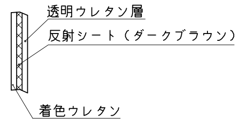
B部詳細図
