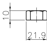
M12ナット
