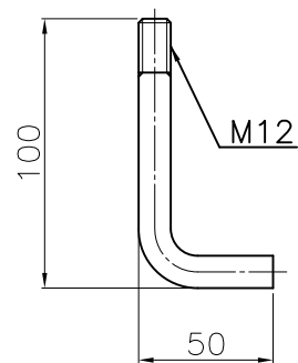
アンカーボルト
