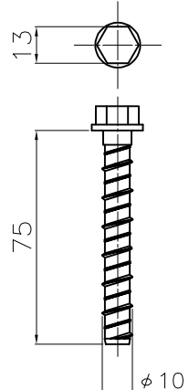
アンカー (4個)
