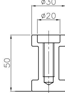
埋設用脚 (4個)
