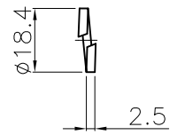
スプリングワッシャ (4個)
