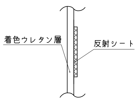
A部詳細断面図
