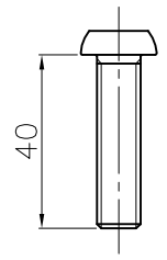
ボルト (M10×1.25P) (4個)
