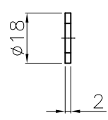
ワッシャ (4個)
