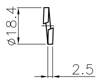
スプリングワッシャ (4個)
