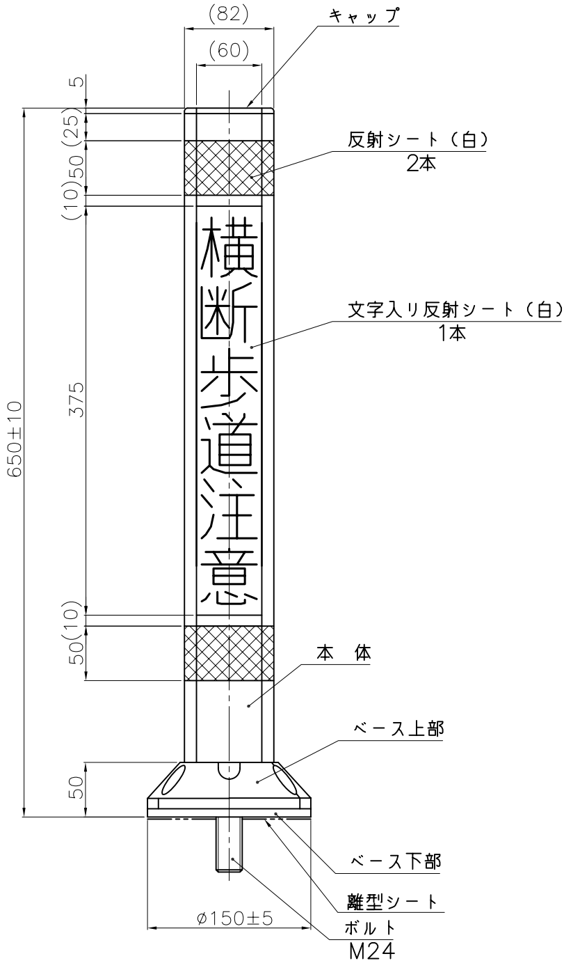
埋設用脚セット図
