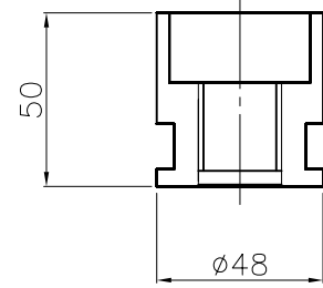
埋設用脚
