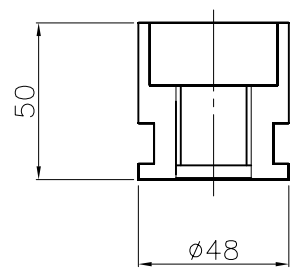
埋設用脚
