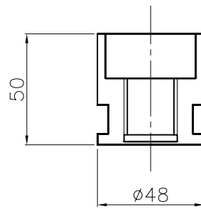
埋設用脚
