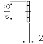
ワッシャ
