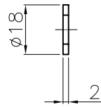
ワッシャ
