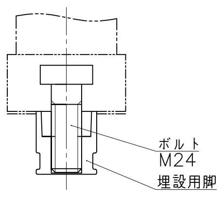
埋設用脚セット図
