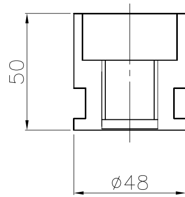
埋設用脚
