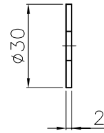
ワッシャ
