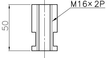
埋設用脚
