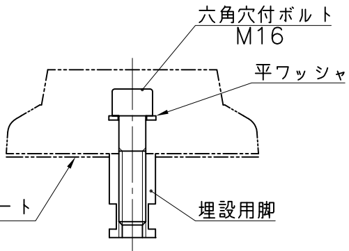
埋設用脚セット図
