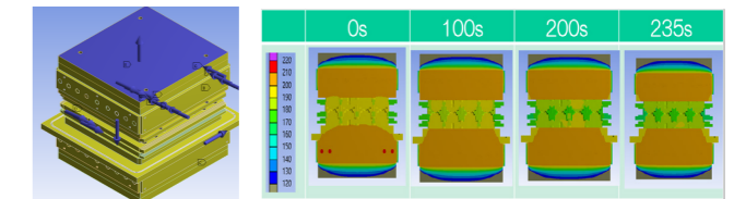
図1. 金型モデル 図2. 製品取り出し時の金型温度変化
