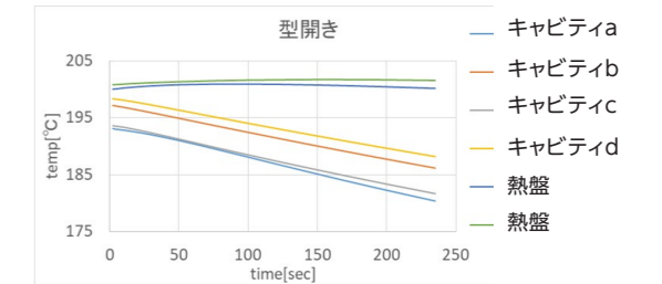
図3. 製品取り出し時の金型内のキャビティの温度変化
