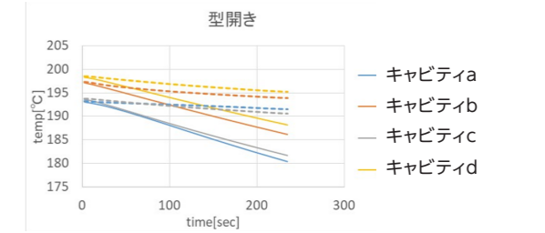
図4. キャビティ温度の変化 実線: 改善前、破線改善後
